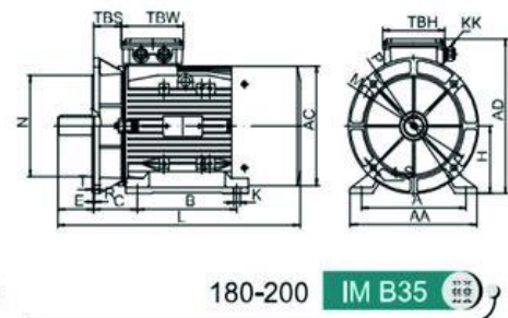
180-200 IM B5
