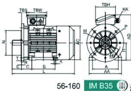
56-160 IM B34
